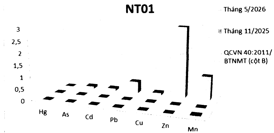
Biểu đồ 7. Diễn biến hàm lượng các kim loại trong nước thải của kho Hải Phòng (tháng 5/2026 và tháng 11/2025)
