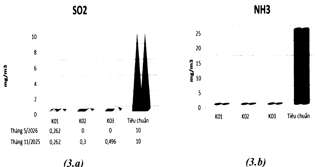
Biểu đồ 3. Diễn biến chất lượng SO 2 (3.a) và NH 3 (3.b) khu vực hoạt động sản xuất của kho Hải Phòng (tháng 5/2026 và tháng 11/2025)
