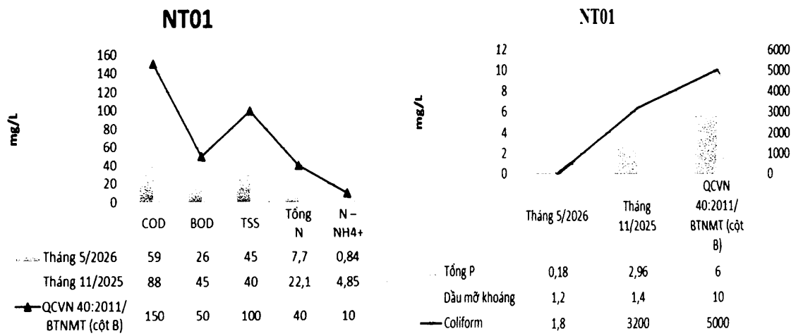
Biểu đồ 6. Diễn biến các thông số hữu cơ và sinh học trong nước thải của kho Hải Phòng (tháng 5/2026 và tháng 11/2025)
